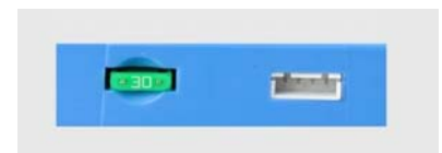
1 PIN:N/A 2 PIN:SMBC 3 PIN:SMBD 4 PIN:GND
